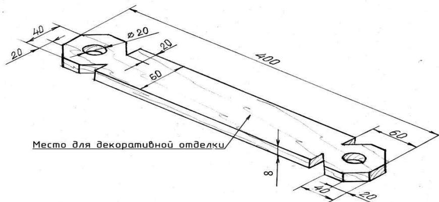
Рис.1 Наличник декоративный
